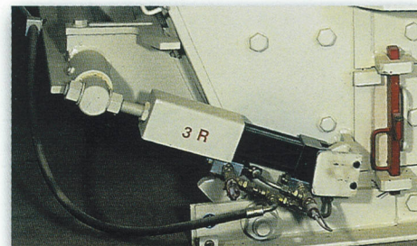
Sistema di regolazione idraulica del portacorazze - optional
